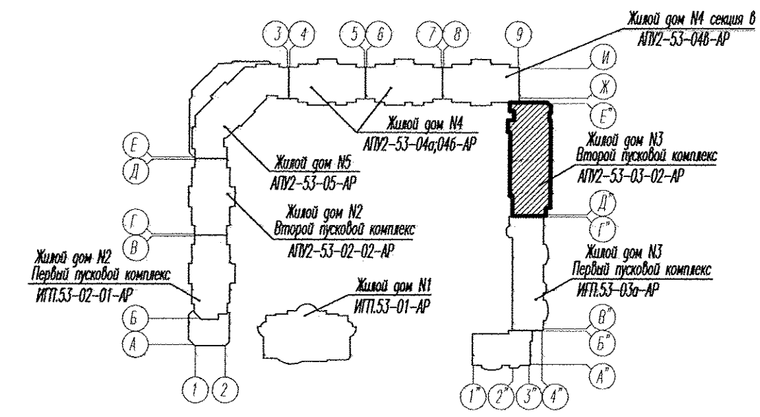
Компоновочная схема
